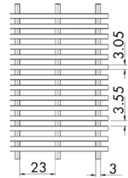
Tile Insert
